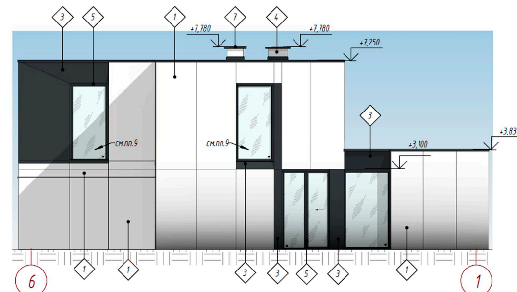
Фасад 6-1
