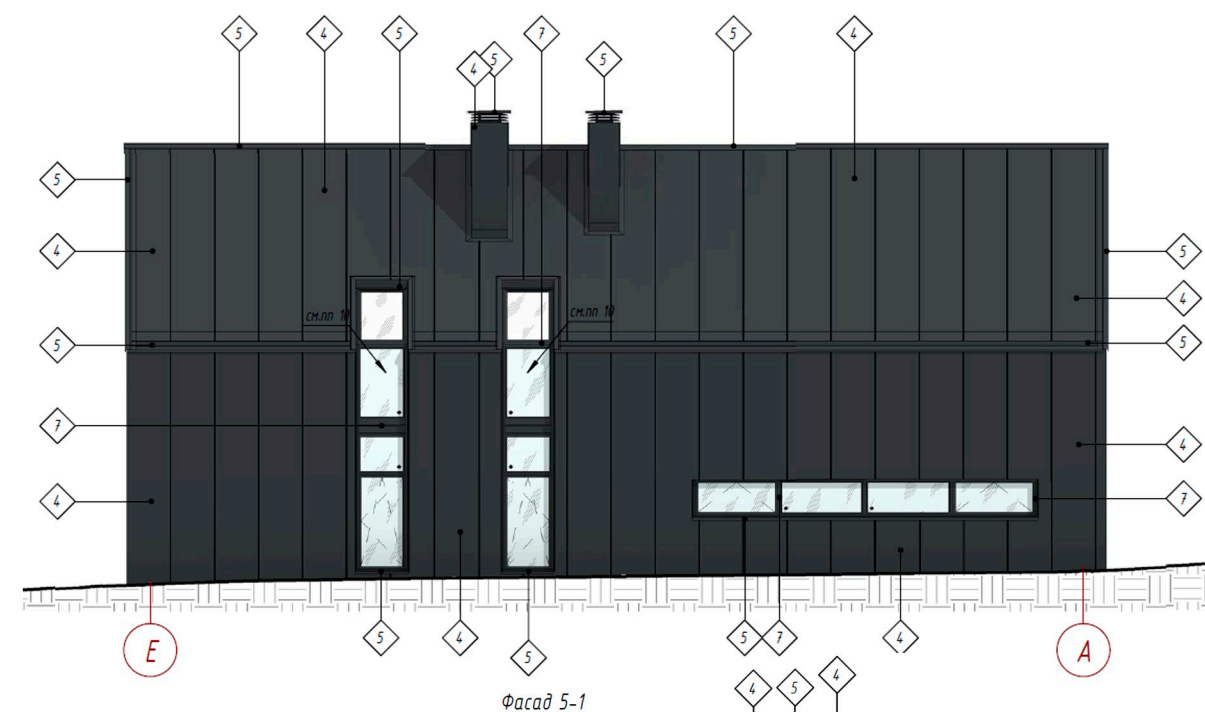
Фасад E-A
