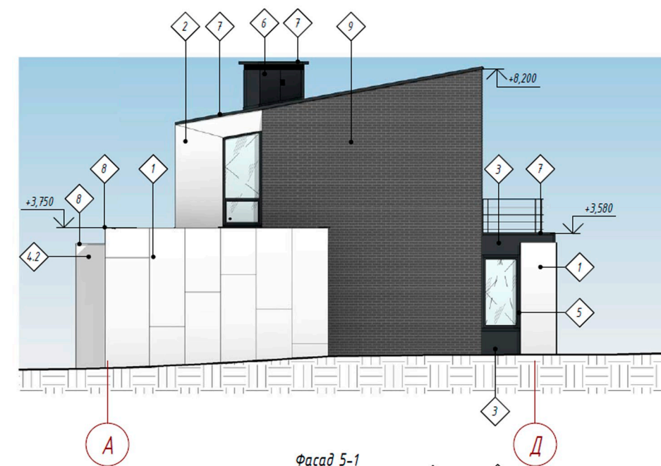
Фасад А-Д
