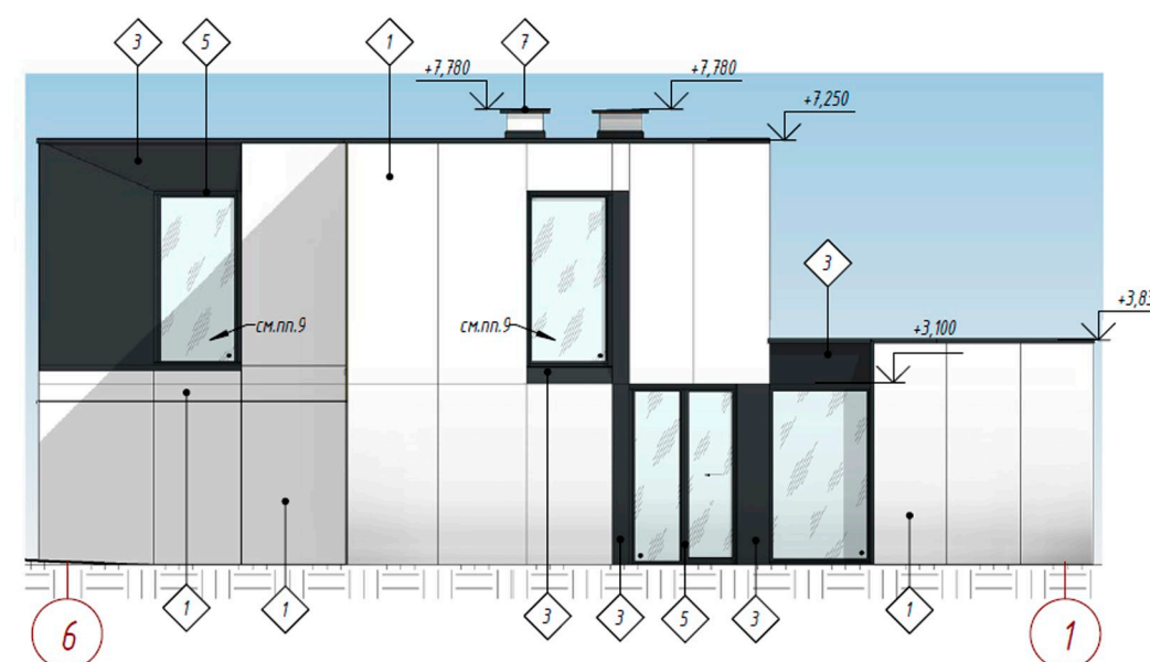
Фасад 6-1
