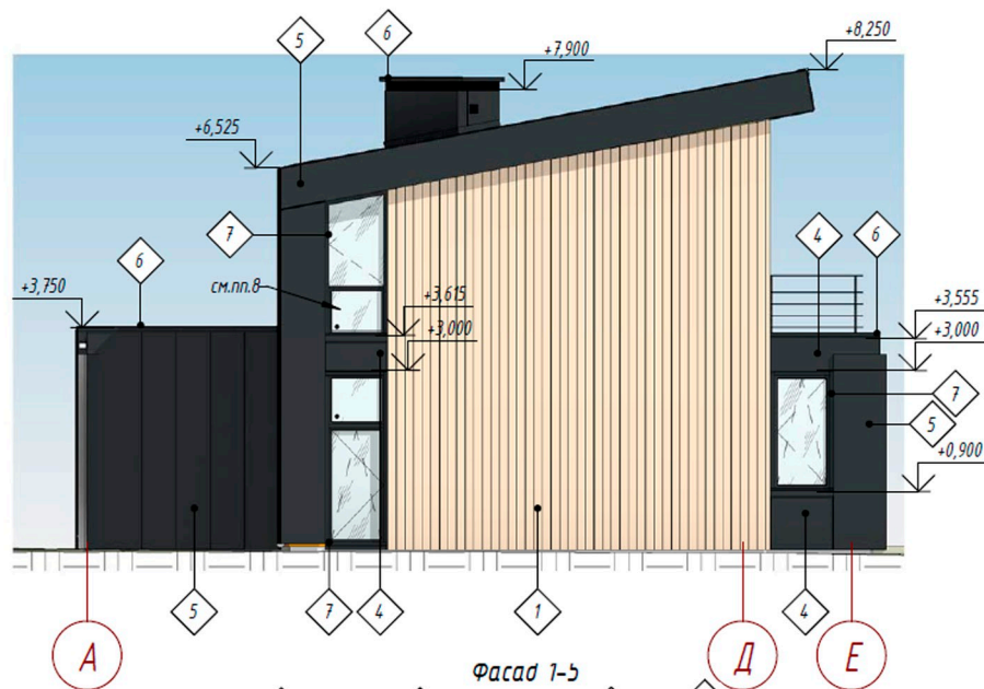
Фасад E-A
