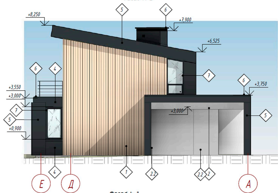
Фасад 5-1
