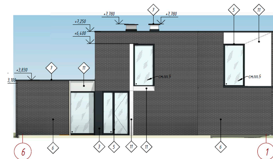
Фасад 6-1
