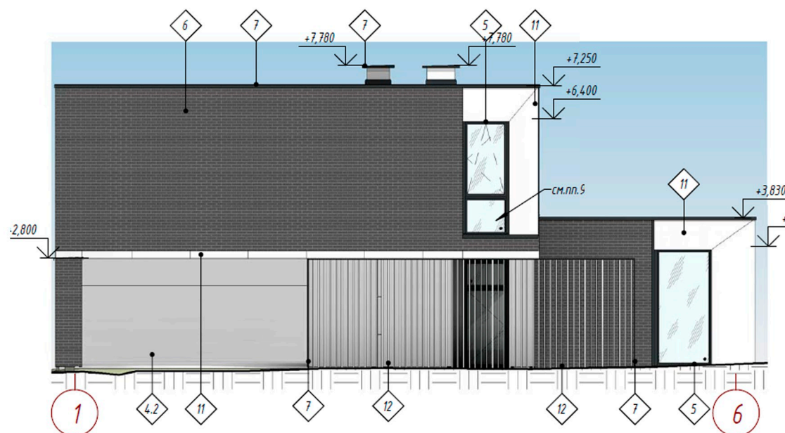
Фасад 1-6
