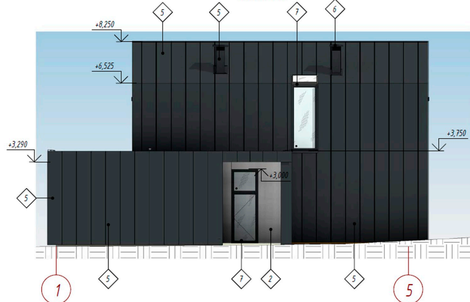
Фасад 1-5
