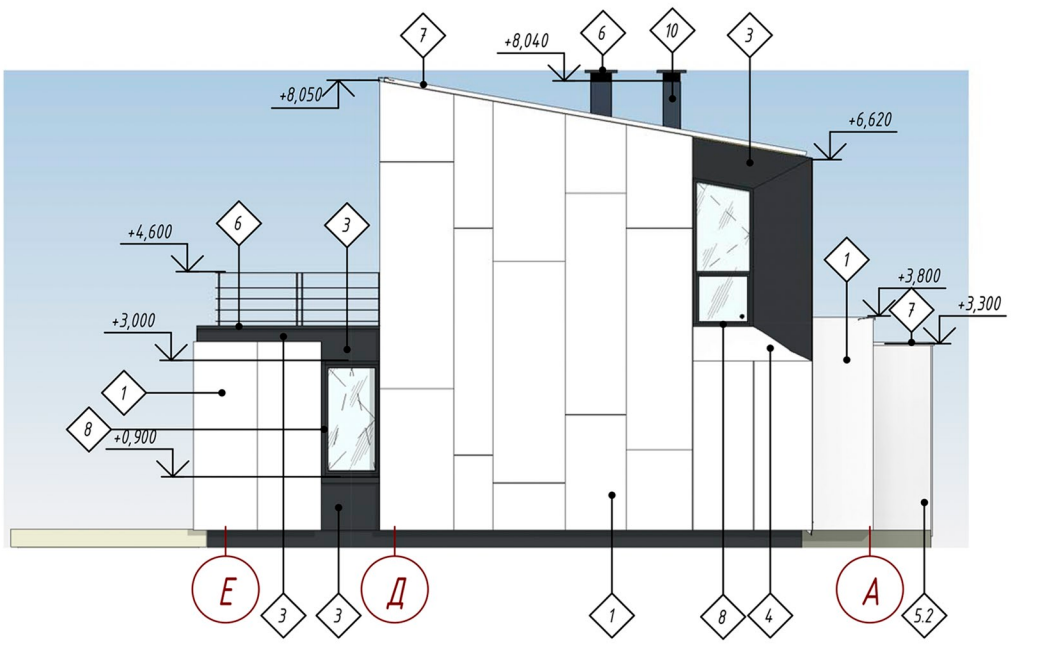
Фасад Е-А
