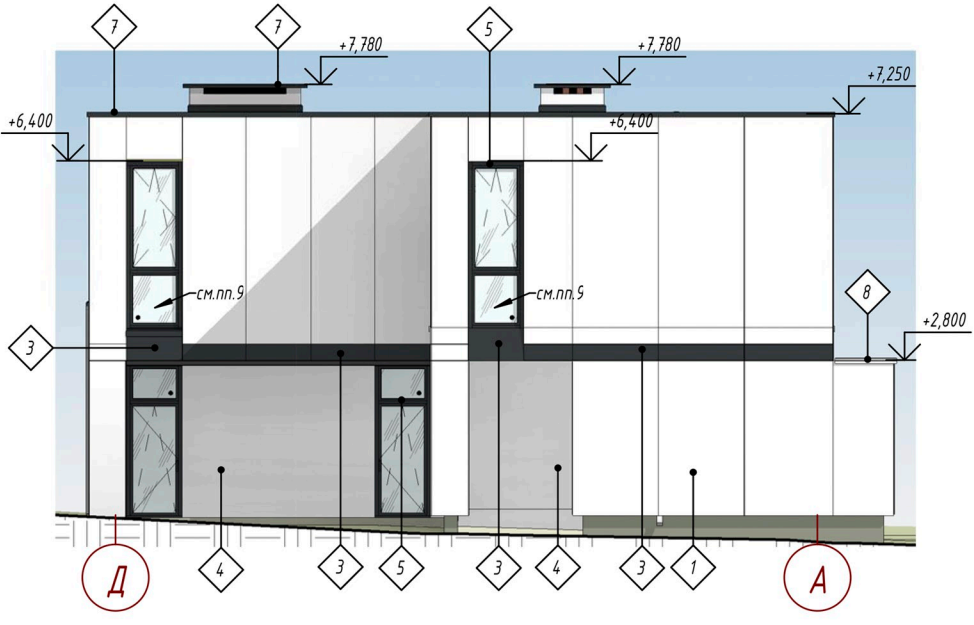
Фасад Д-А
