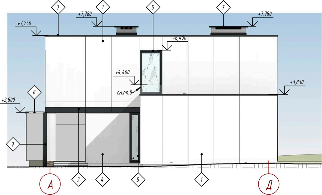
Фасад А-Д
