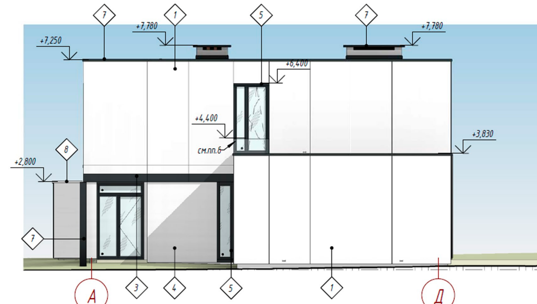
Фасад А-Д
