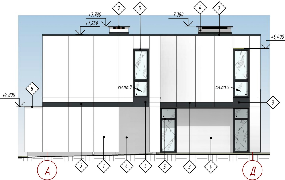
Фасад А-Д
