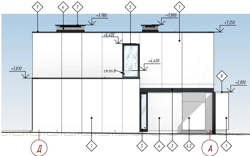
Фасад Д-А
