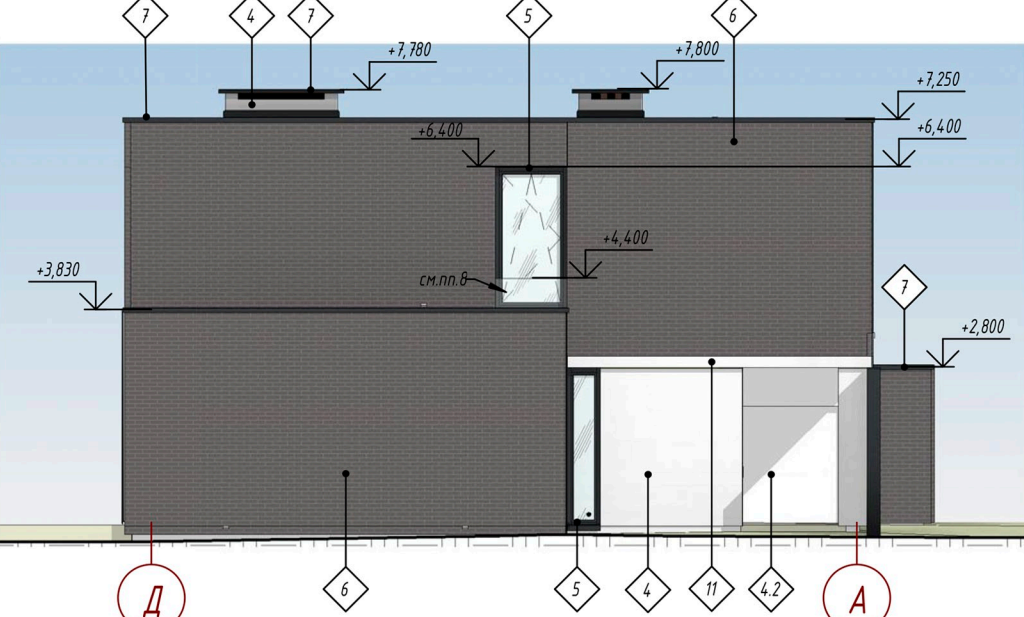
Фасад Д-А
