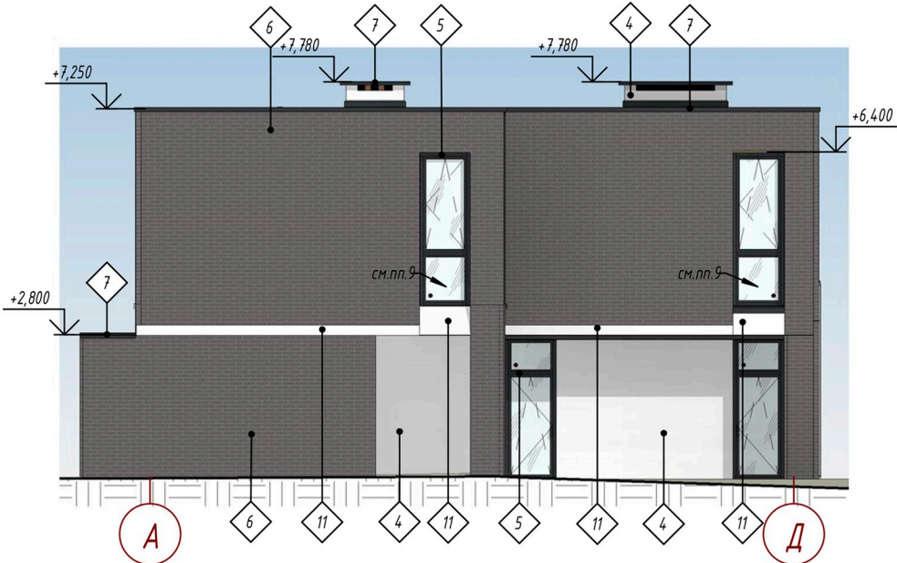
Фасад А-Д
