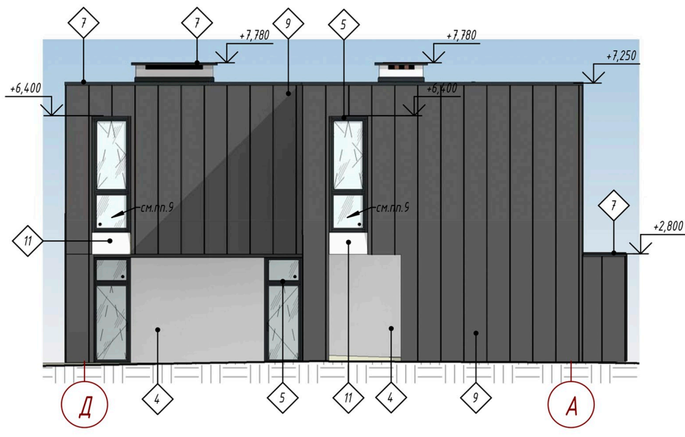
Фасад Д-А
