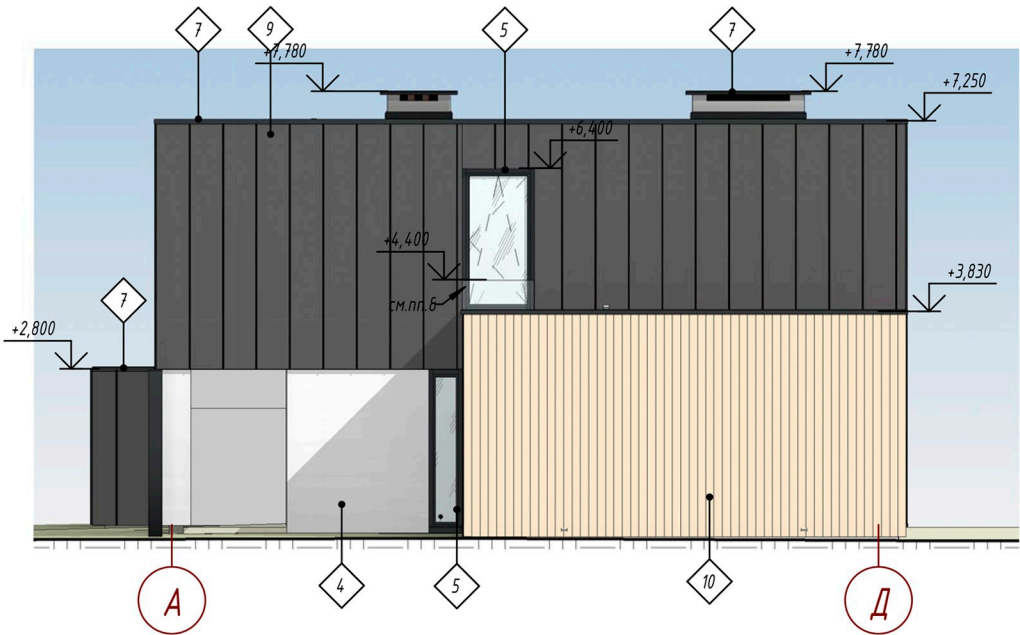
Фасад А-Д
