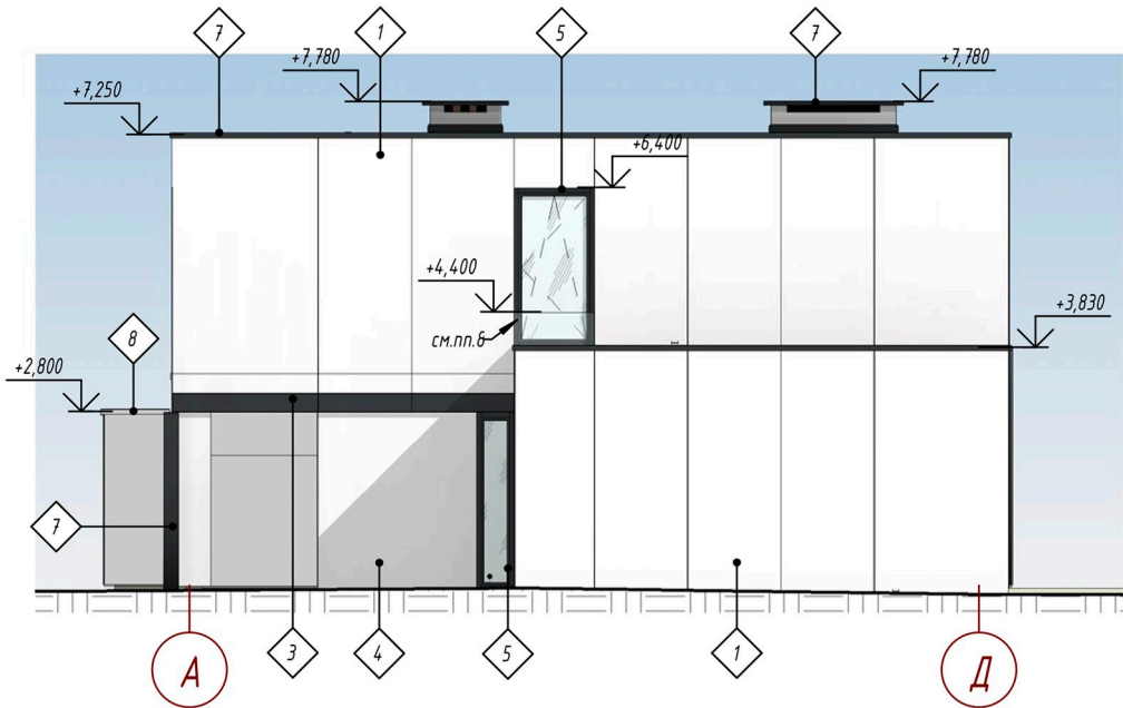
Фасад А-Д
