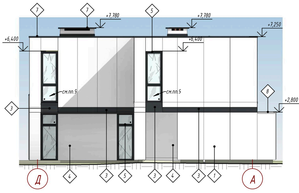
Фасад Д-А
