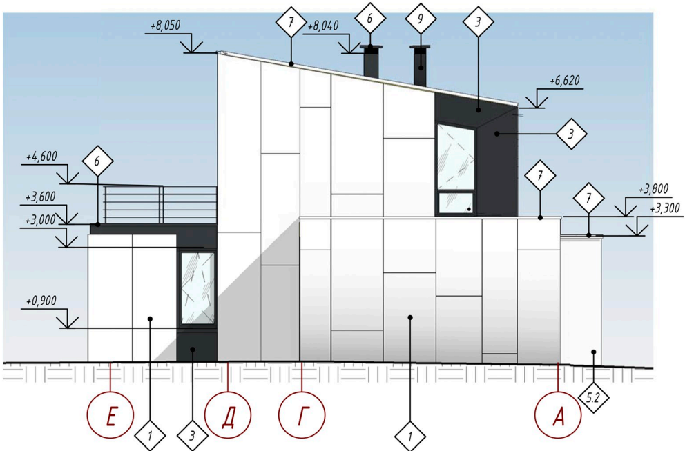
Фасад Е-А
