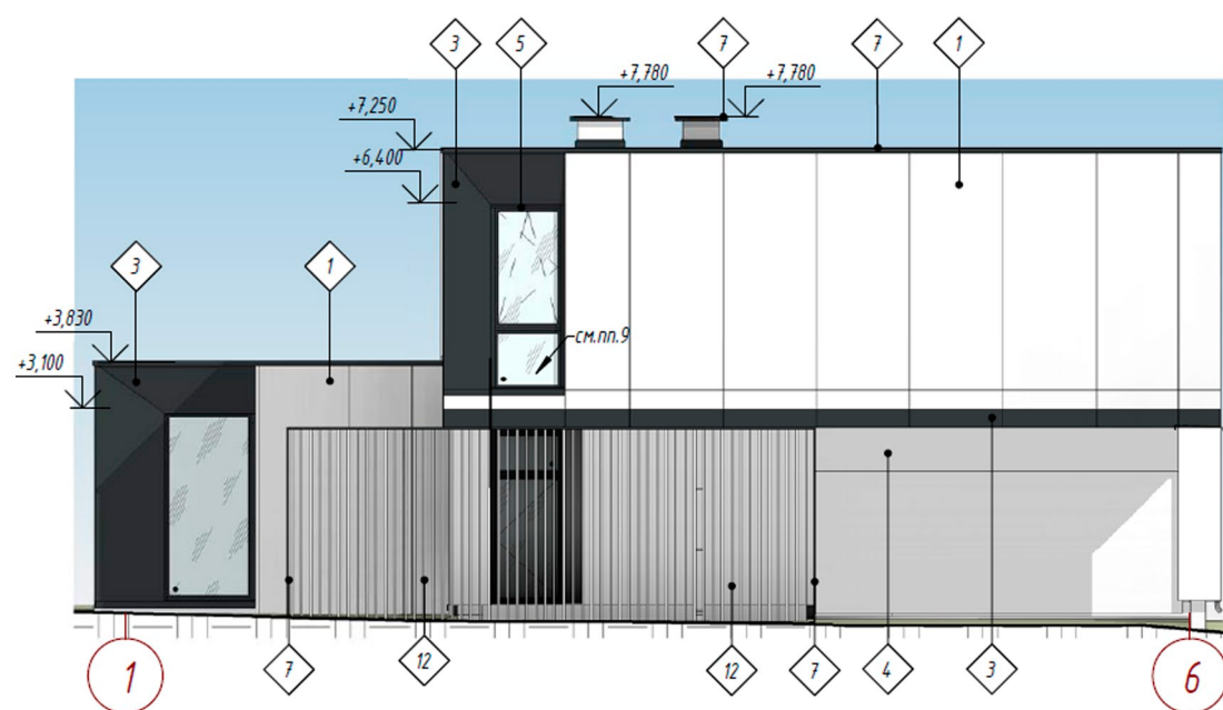
Фасад 1-6
