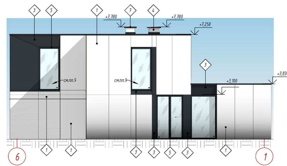
Фасад 6-1
